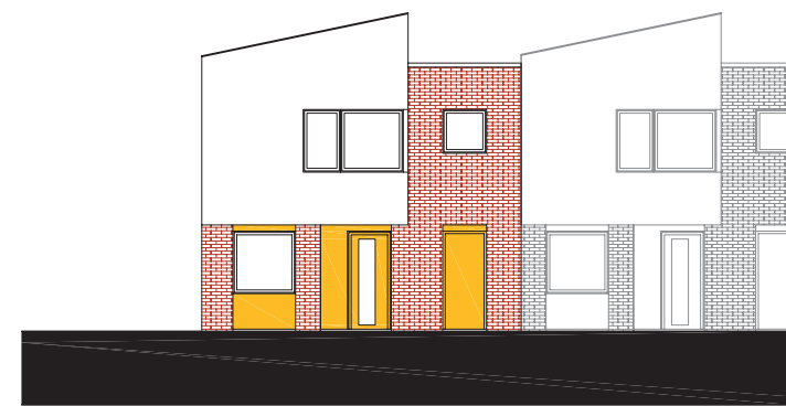
POHLED 1
