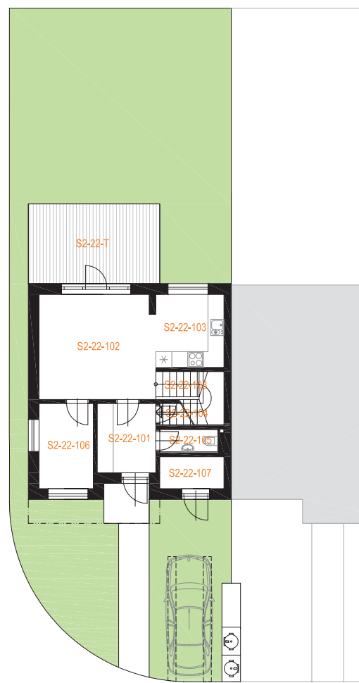
PŮDORYS 1.NP
